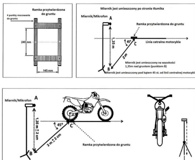
Rys. nr. 1 - Umieszczenie miernika głośności względem motocykla
