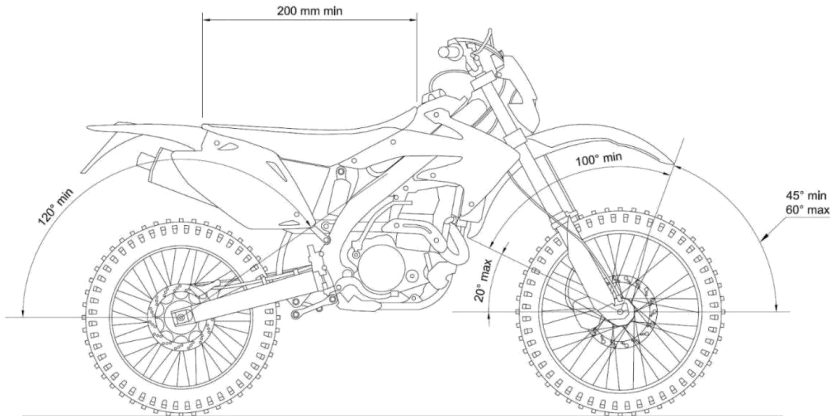
Rys. nr. 2 - motocykl enduro - widok z boku
